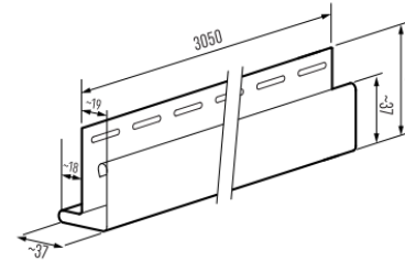
SV (P) 12.5 Outside corner mini
