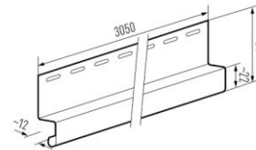
SV(P) 16.5 Drip edge
